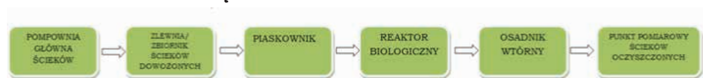
Schemat Oczyszczalni Ścieków w Dębem Wielkim:
