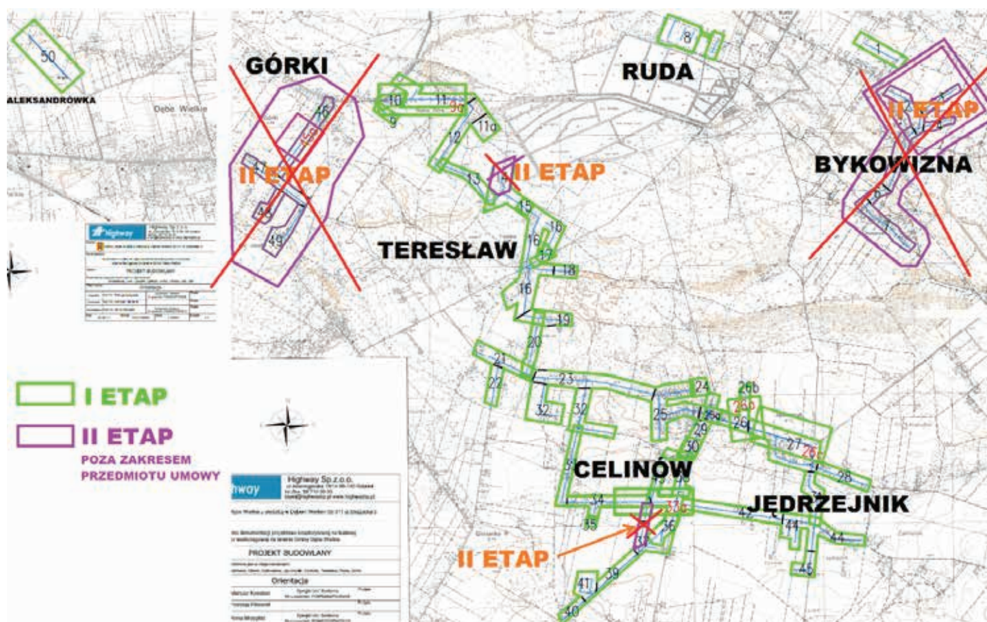
Zakres zleconych prac budowy sieci wodociągowej
